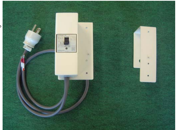
写真は基本ベース 1台用シーケンサCPU取付金具
